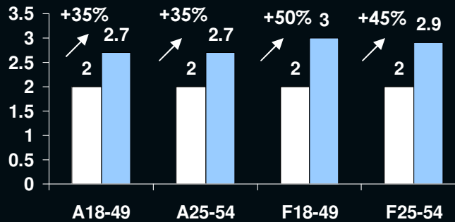
Vancouver EM
