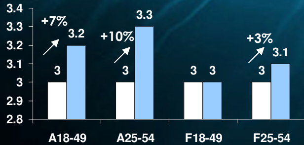
Toronto EM
