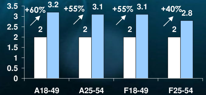
Calgary EM
